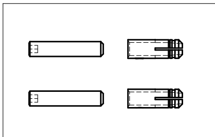
M6 Befestigungsset 266.050.004
