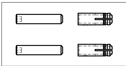
M6 Befestigungsset 266.050.004
