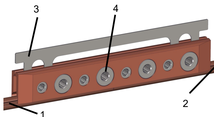
B: Griffe striée avec plaque d'écartement en acier pour la rainure du fil de contact type BC, Rainure du fil de contact 6.78 - 6.90 mm
