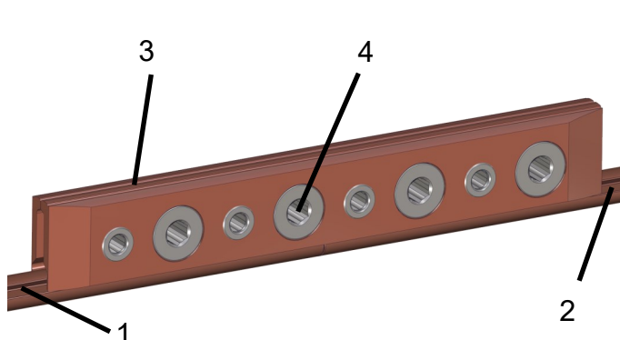
A Griffe striée pour la rainure du fil de contact type AC, Rainure du fil de contact 5.51 - 5.60 mm
